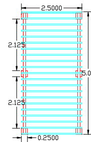
PLANTA BAIXA ESCALA 1:100
